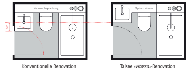
«vitessa» wird direkt an die bestehende Wand befestigt. Auf eine vorgebaute Wand wird verzichtet. Dadurch gewinnt man bis zu 20 cm Wohnraum im Bad im Vergleich zu einer konventionellen Renovation.
